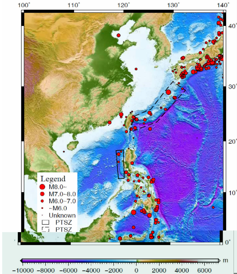
图 1 我国东部及近海邻国引发海啸的强震分布图
