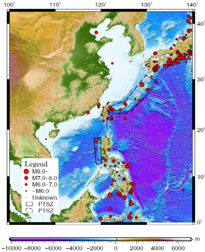
图 1 我国东部及近海邻国引发海啸的强震分布图
